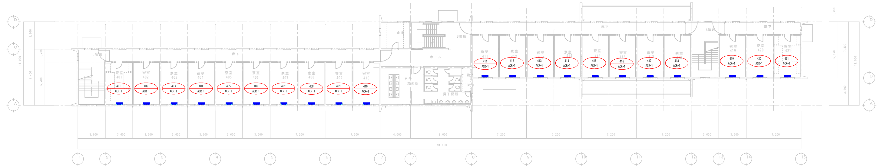
生徒寄宿舎4階 S=1/150
