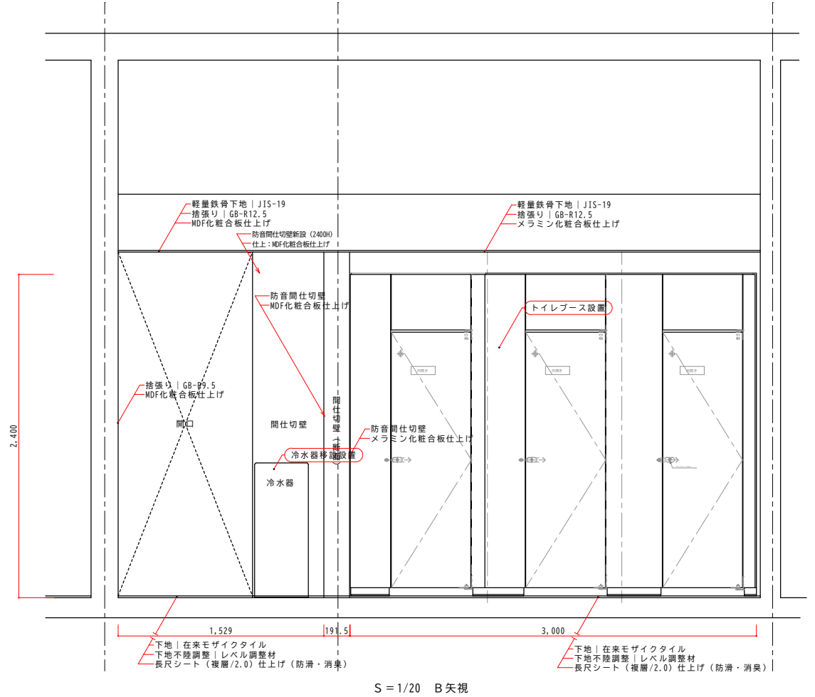
S=1/20 B矢視
