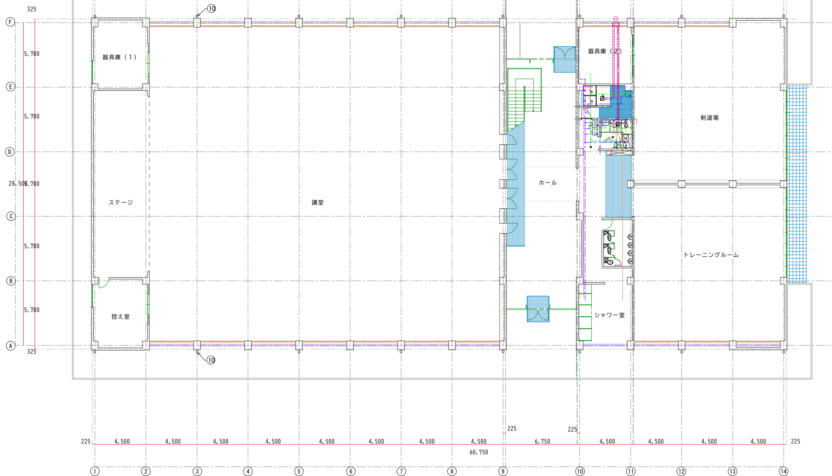
在来 1階平面図 S=1/100
