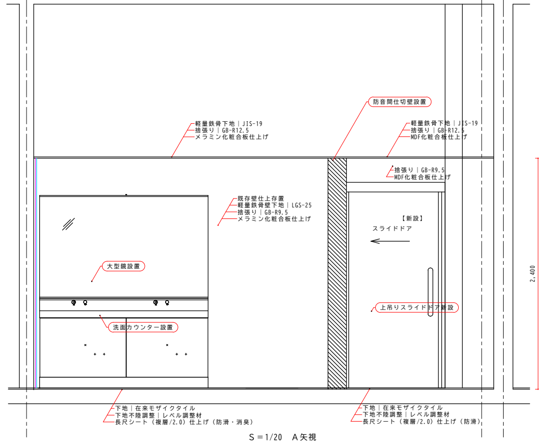
S=1/20 A矢視
