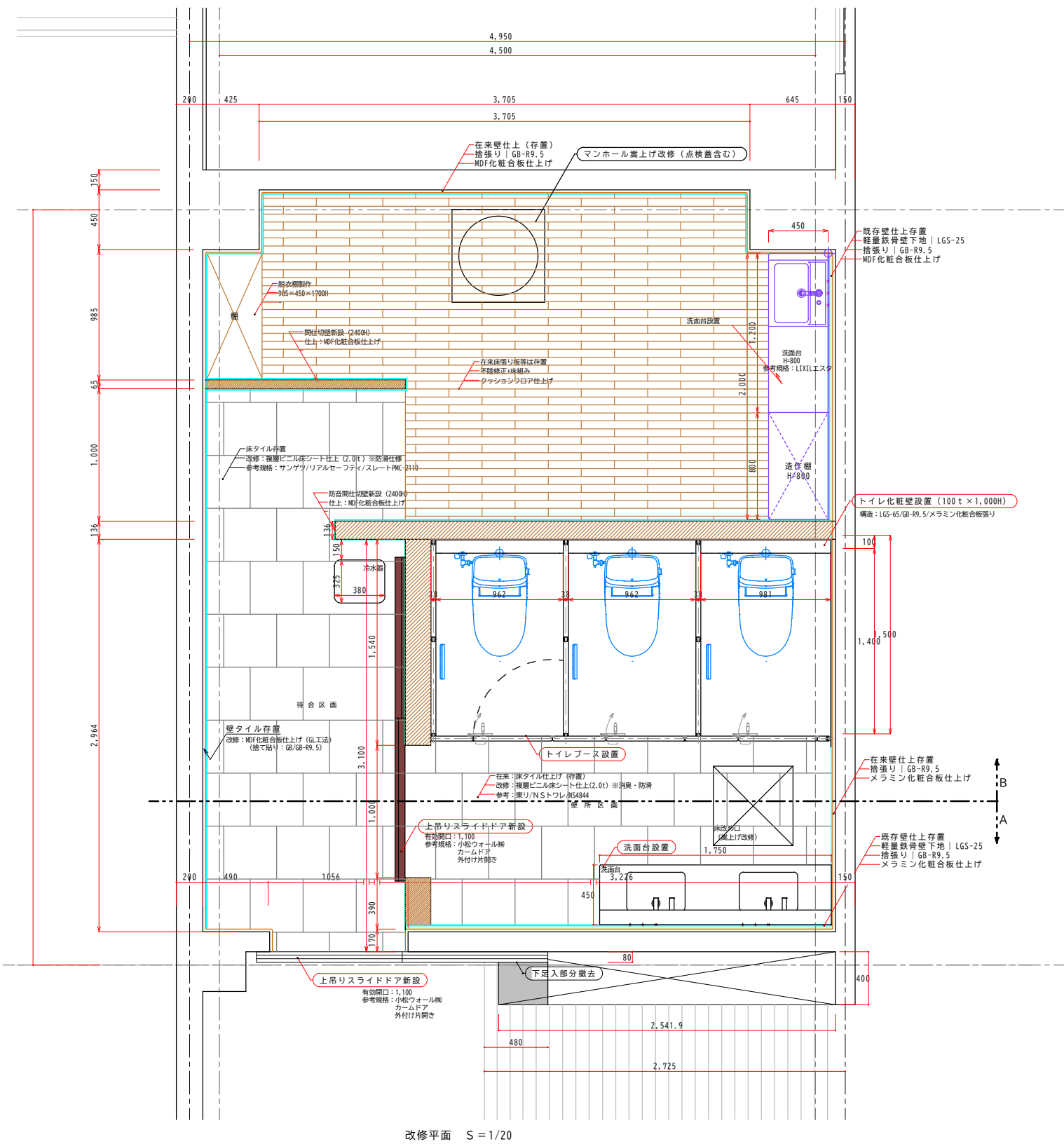
改修平面 S=1/20
