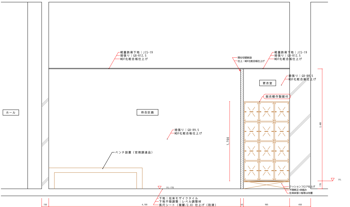
S=1/20 F 矢視
